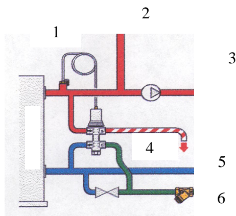
Joonis 2. Kaitseklapi ühendamine
